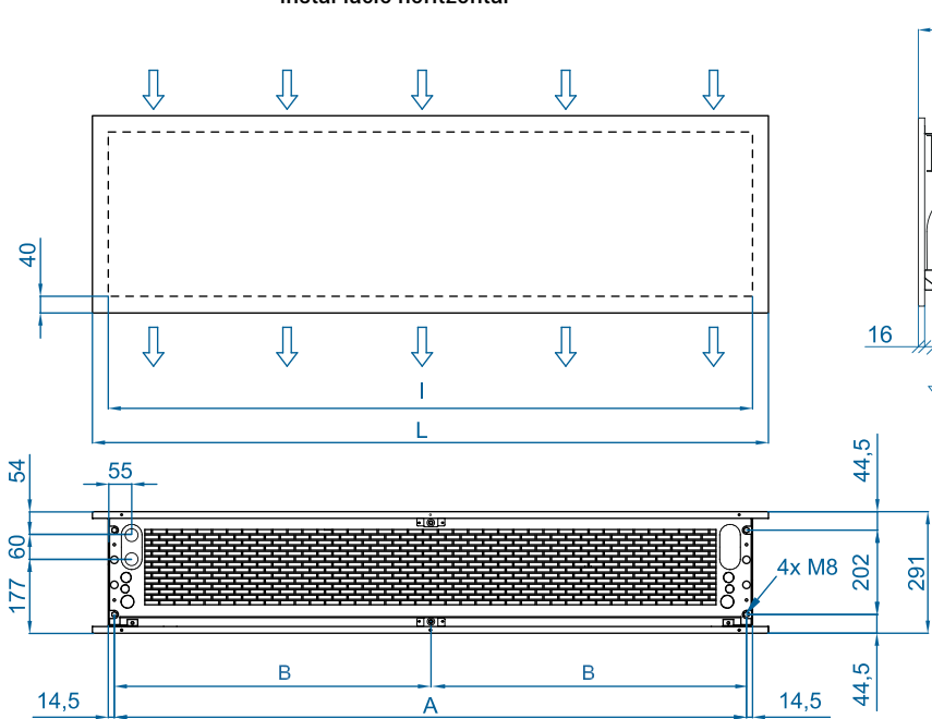
Instal·lació horitzontal
