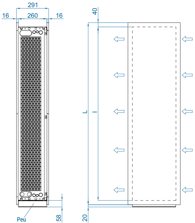
Instal·lació vertical
